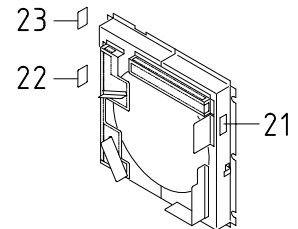
FAN SHROUD
